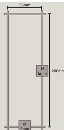
Maille du panneau Aquilon® 55 Medium
